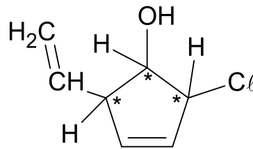
2-cloro-5-vinilciclopent-3-en-1-ol
